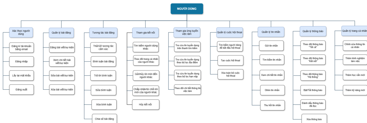
Hình 2.3: Sơ đồ phân rã chức năng của User ( Link )
