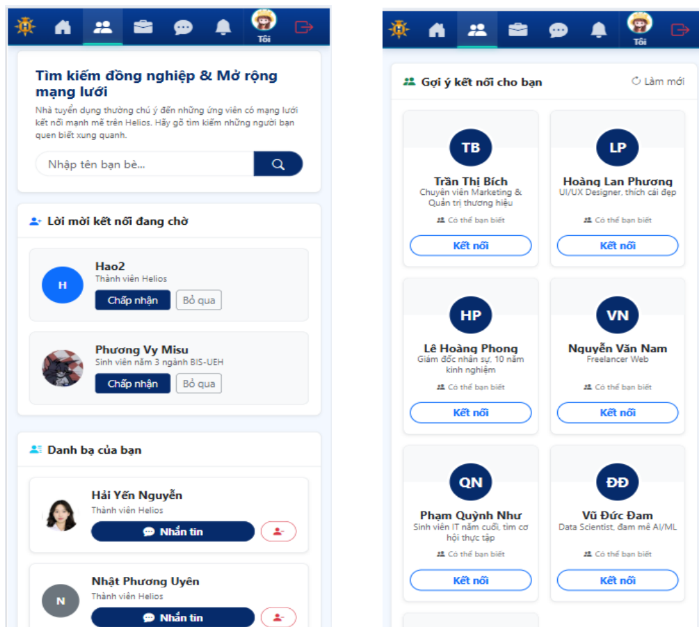
Hình 3.13: Giao diện Mạng lưới hiển thị trên mobile
