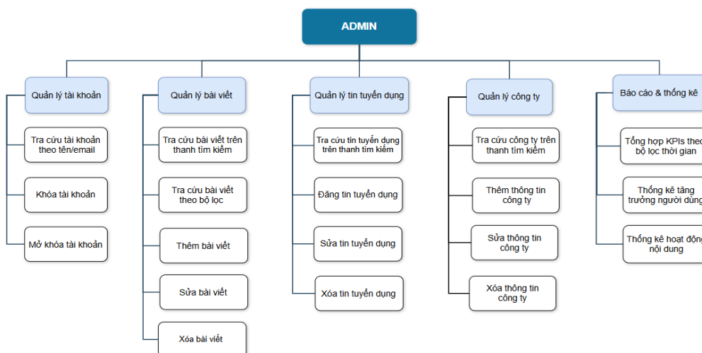
Hình 2.2: Sơ đồ phân rã chức năng của Admin ( Link )
