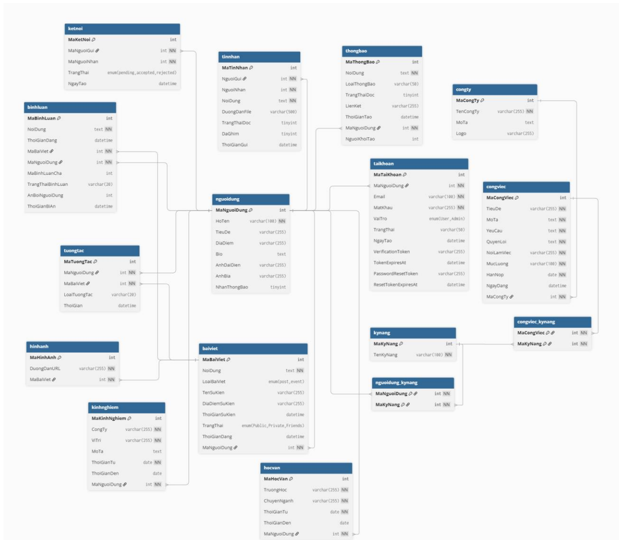
Hình 4.1: Sơ đồ quan hệ ERD ( Link )
