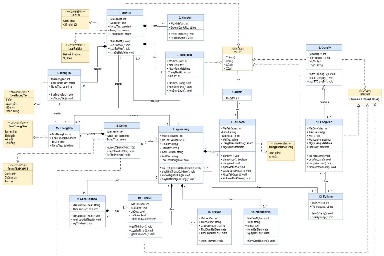
Hình 2.4: Sơ đồ lớp Class Diagram ( Link )
