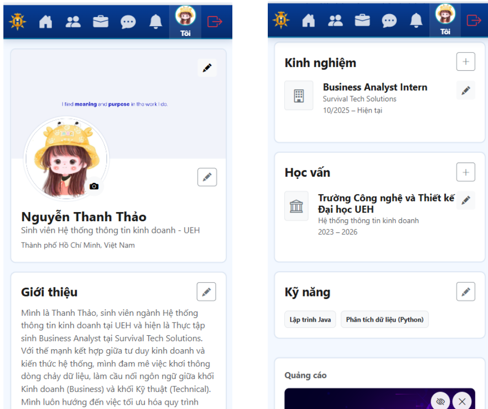
Hình 3.25: Giao diện trang Cá nhân hiển thị trên mobile
