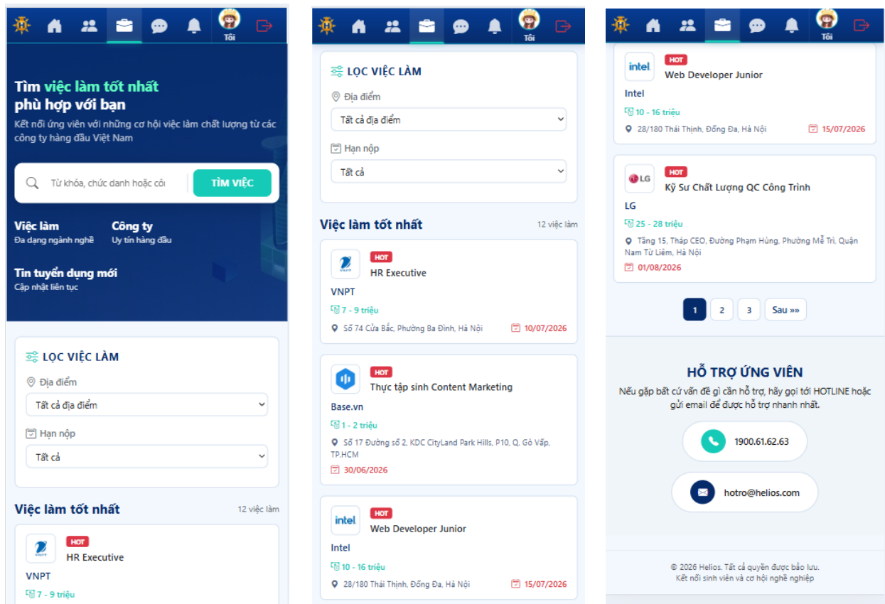
Hình 3.17: Giao diện Việc làm hiển thị trên mobile
