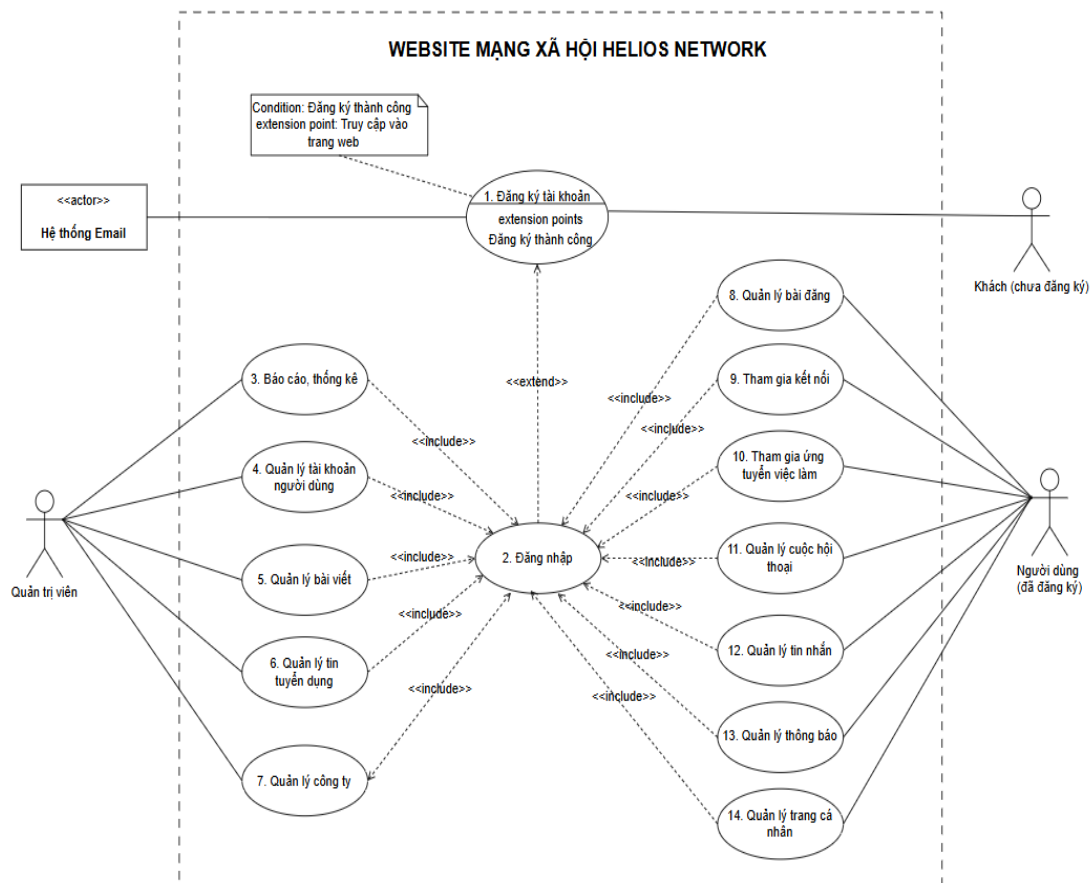
Hình 2.1: Sơ đồ Use Case tổng quát ( Link )
